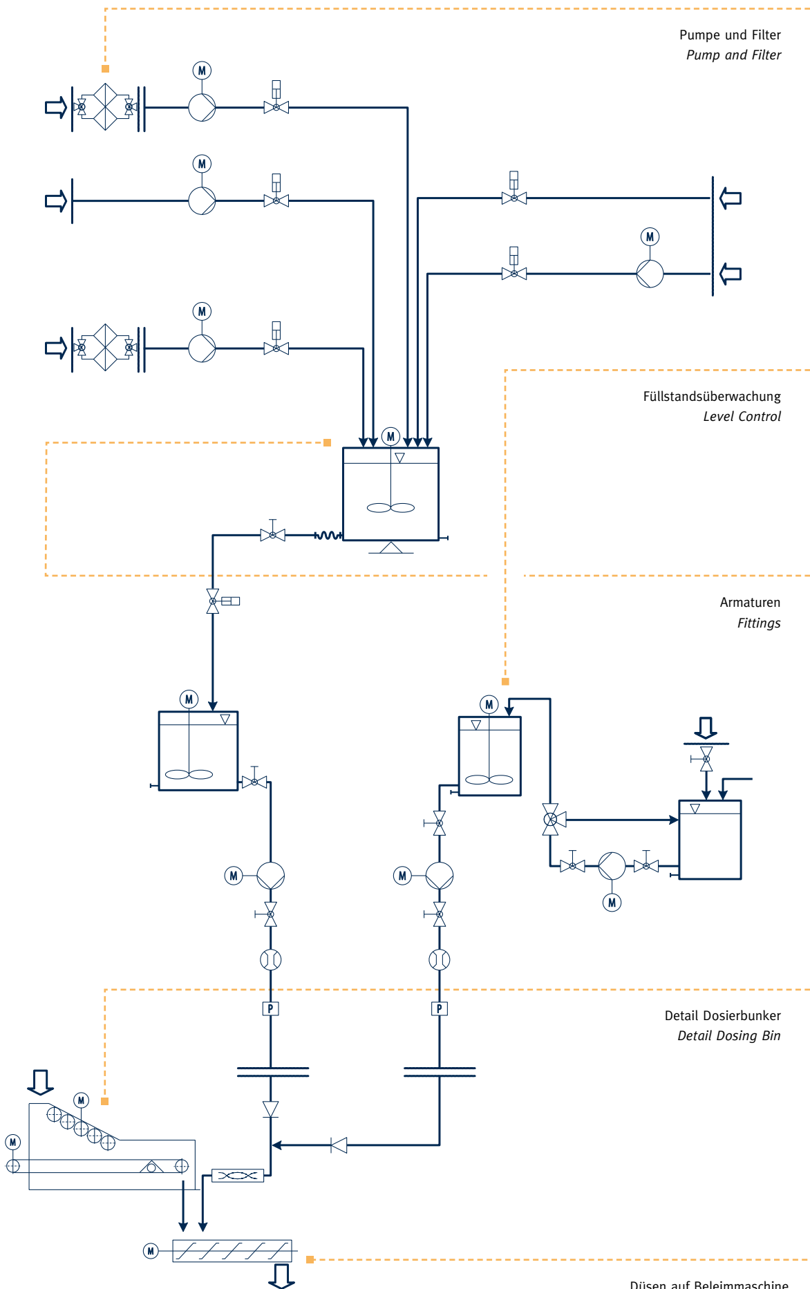
Düsen auf Belemmaschine Nozzles on Glue Blender
