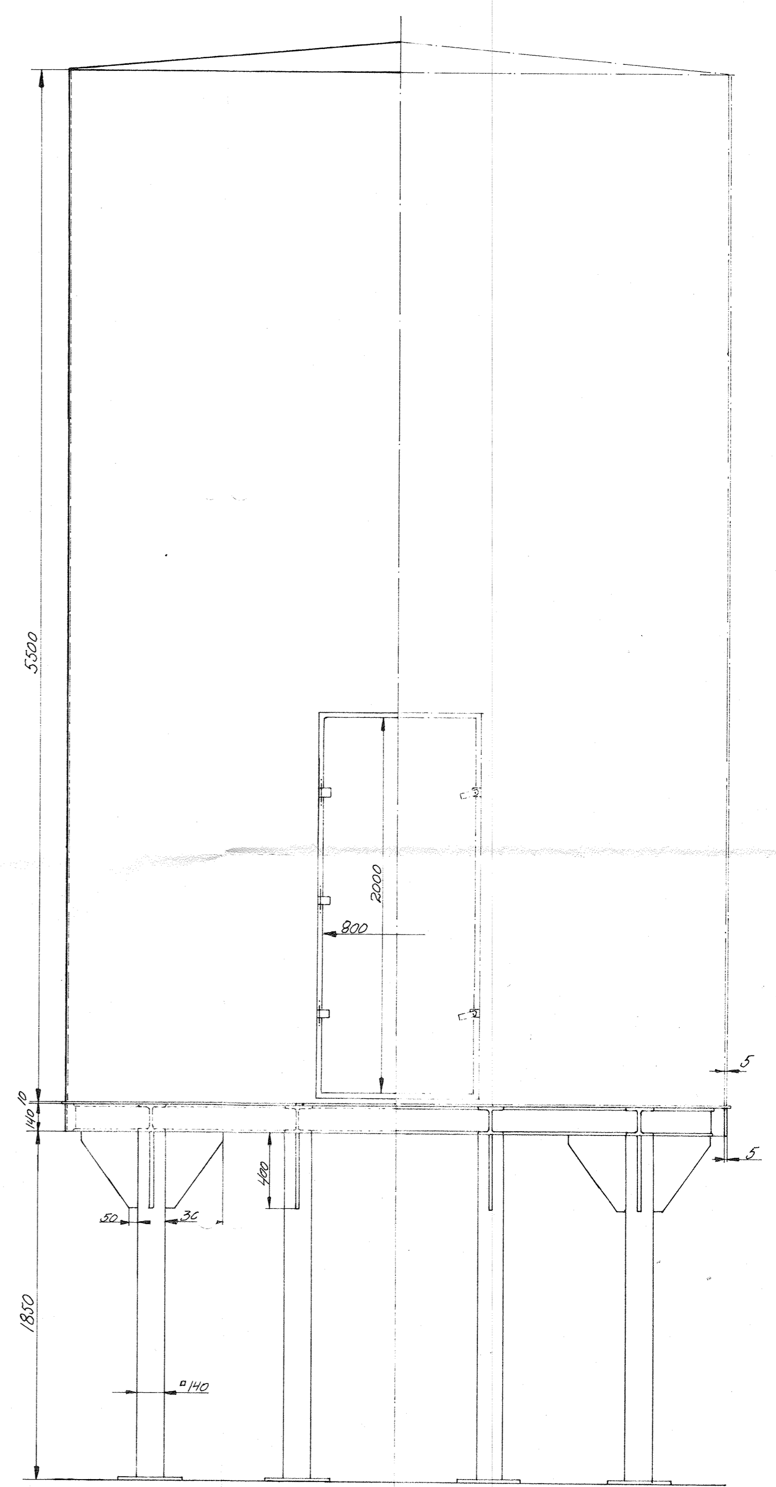
SCHNITT B-B
